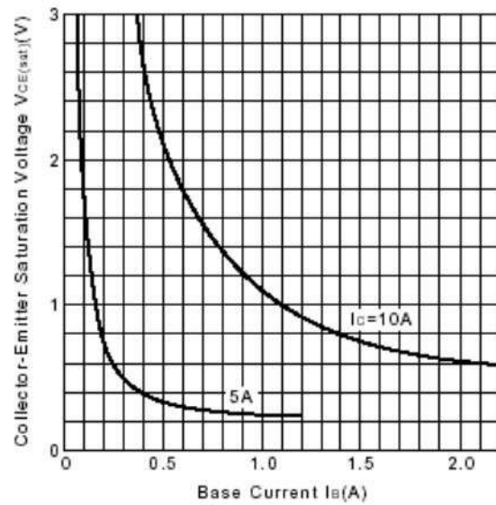
Fig.4 V_{CE(sat)} - I_B
