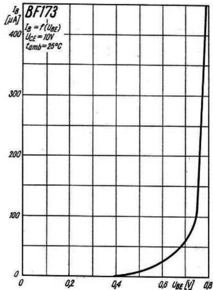
Rys. 1-456. Charakterystyka wejściowa
