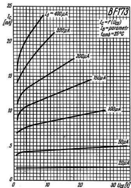
Rys. 1-455. Charakterystyki wyjściowe
