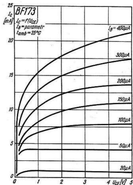
Rys. 1-454. Charakterystyki wyjściowe
